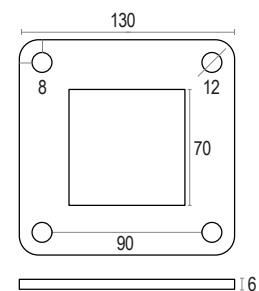
Piastra della colonna in alluminio
