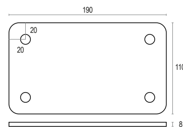
Piastra tassellare per recinzioni H 1600 - 1800 - 2000
