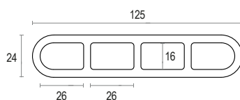
Doga per staccionata con profilo quadro
