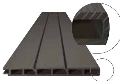
Doga terminale smussata Chiude la recinzione in altezza
