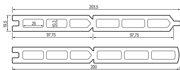
Doghe coestruse Normale e smussata
