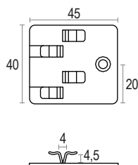
Clip per rivestimento Classic inox doppio uso AF611
