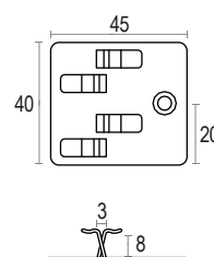
Clip per pavimento Professional doppio uso
