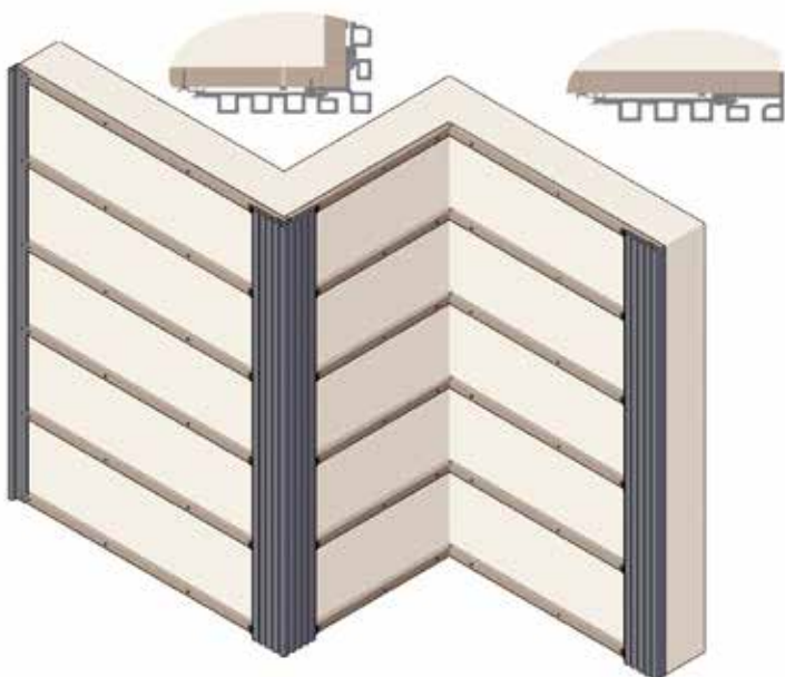
Iniziare l'installazione del rivestimento.
