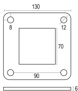
Piastra della colonna in alluminio
