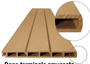
Doga terminale smussata Chiude la recinzione in altezza
