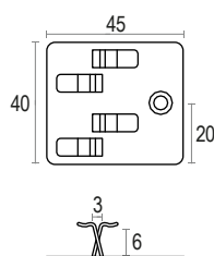
Clip per pavimento Classic doppio uso
