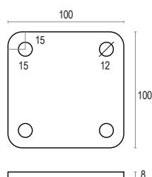
Piastra tassellare per recinzioni H 1000 - 1200 - 1400
