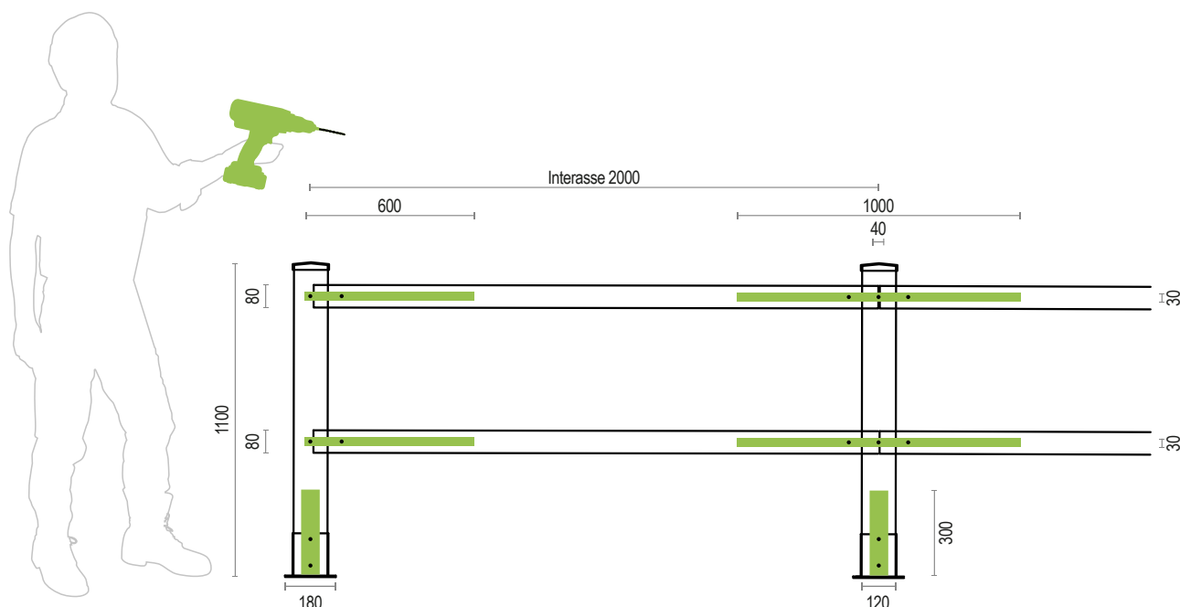
Colonna di partenza
